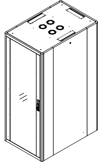
İzometrik Görünüş
