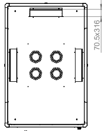
Üst Görünüş
