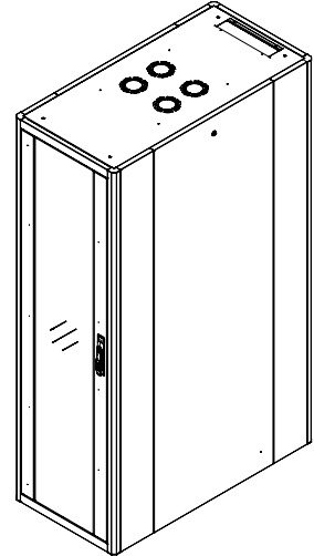
İzometrik Görünüş
