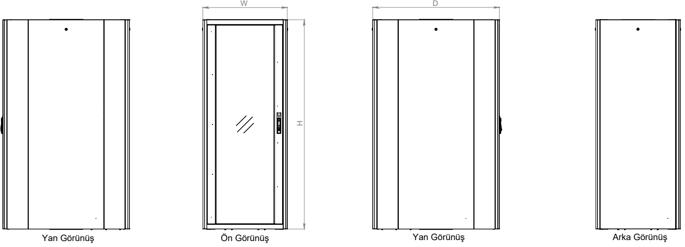
Yan Görünüş
