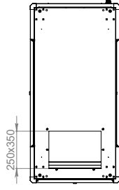
Alt Görünüş
