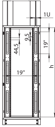
ÖN KAPAKSIZ GÖRÜNÜŞ
