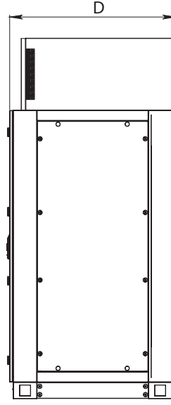
YAN GÖRÜNÜŞ
