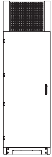
ARKA GÖRÜNÜŞ
