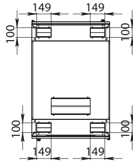
ALT GÖRÜNÜŞ
