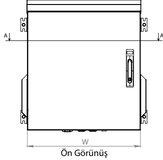
Ön Görünüş
