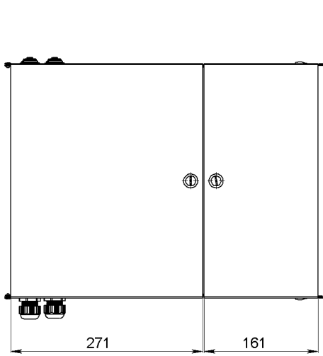
Ön Görünüş
