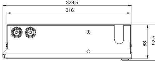
Üst Görünüş
