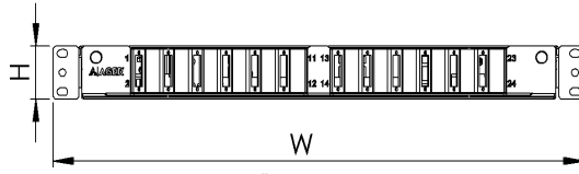
Ön Görünüş
