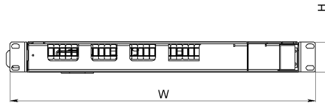
Ön Görünüş
