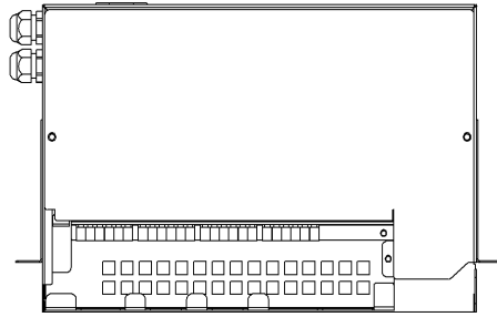
Üst Görünüş
