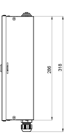
Yan Görünüş
