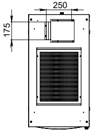
ÜST GÖRÜNÜŞ
