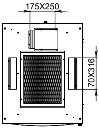
ÜST GÖRÜNÜŞ
