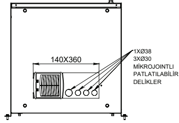
Alt Görünüş
