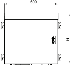
Ön görünüş
