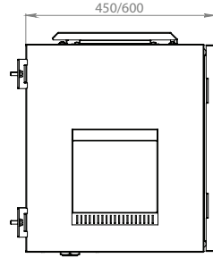
Yan Görünüş
