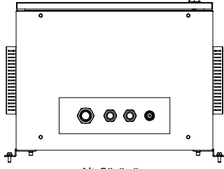
Alt Görünüş
