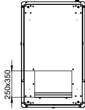
ALT GÖRÜNÜŞ
