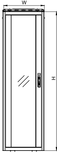
ÖN GÖRÜNÜŞ
