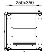
ALT GÖRÜNÜŞ
