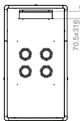
Üst Görünüş
