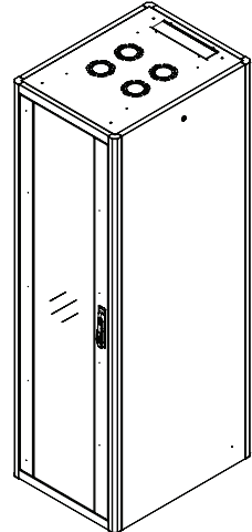
İzometrik Görünüş
