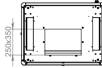
Alt Görünüş
