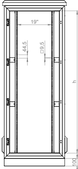
Ön Görünüş
