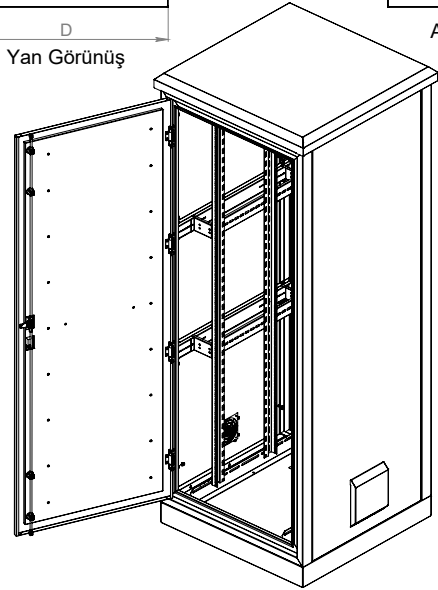
İzometrik Görünüş
