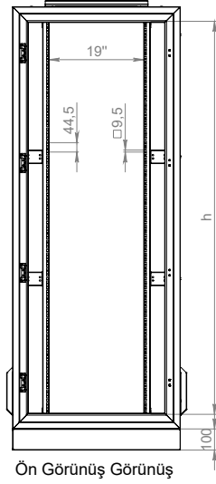
Ön Görünüş Görünüş
