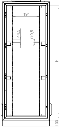
Ön Görünüş
