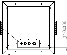
Alt Görünüş
