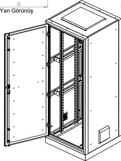
İzometrik Görünüş
