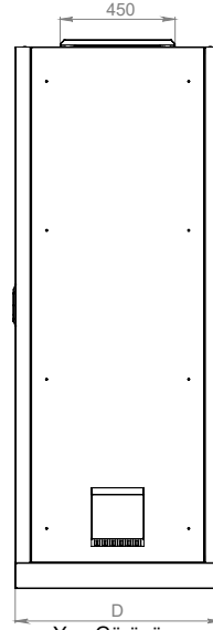
Yan Görünüş
