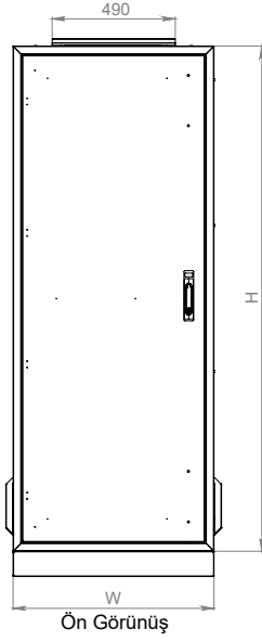
Ön Görünüş
