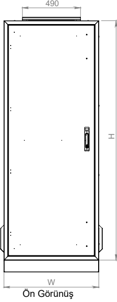
Ön Görünüş
