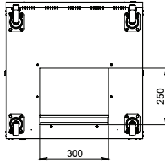
Alt Görünüş
