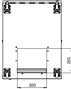
Alt Görünüş
