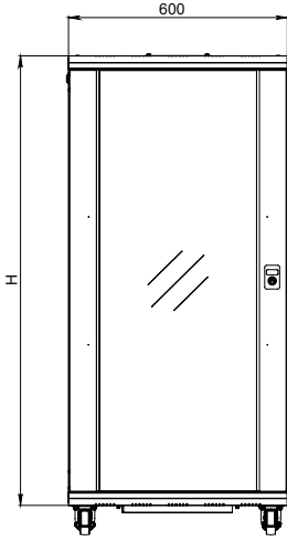
Ön görünüş
