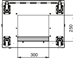
Alt Görünüş
