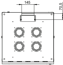
Üst Görünüş
