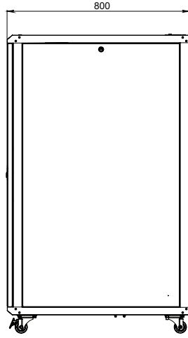
Yan görünüş
