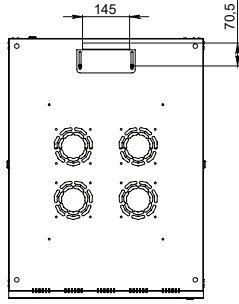
Üst Görünüş
