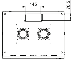
Ön görünüş
