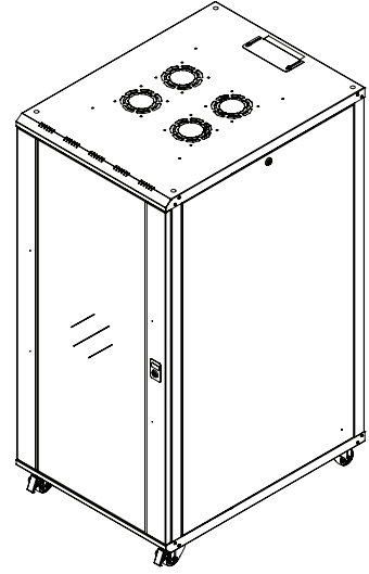
İzometrik görünüş
