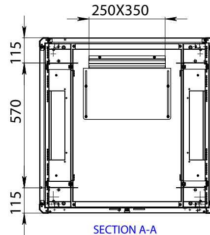
SECTION A-A SCALE 1 : 17
