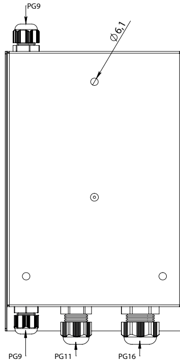
ALT GÖRÜNÜŞ
