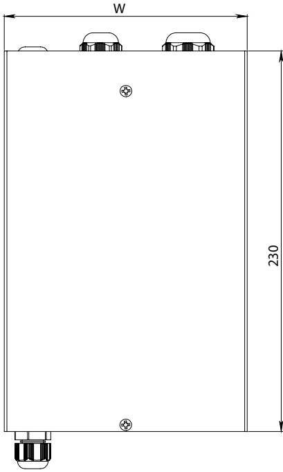
ÜST GÖRÜNÜŞ
