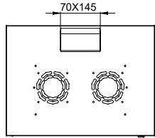
ÜST GÖRÜNÜŞ
