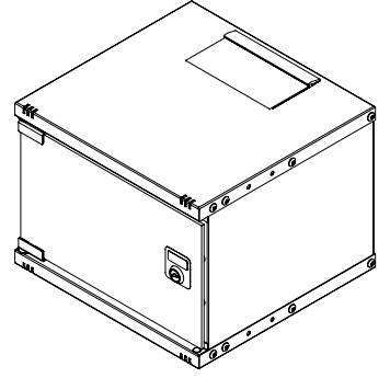
İZOMETRİK GÖRÜNÜŞ
