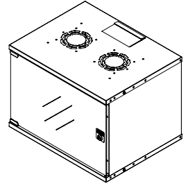
İZOMETRİK GÖRÜNÜŞ
