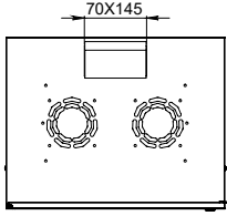
ÜST GÖRÜNÜŞ
