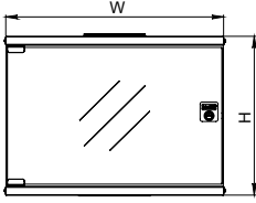
ÖN GÖRÜNÜŞ
