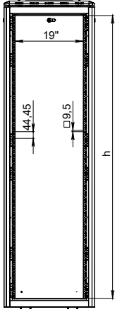
ÖN KAPAKSIZ GÖRÜNÜŞ
