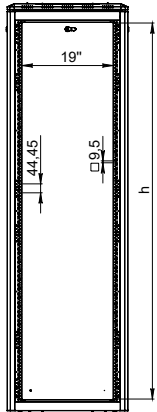
ÖN KAPAKSIZ GÖRÜNÜŞ
