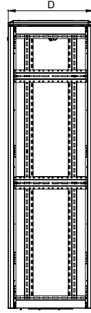
YAN KAPAKSIZ GÖRÜNÜŞ
