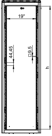
ÖN KAPAKSIZ GÖRÜNÜŞ
