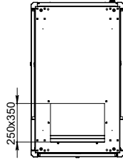
ALT GÖRÜNÜŞ
