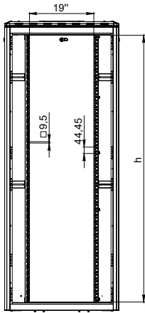
ÖN KAPAKSIZ GÖRÜNÜŞ
