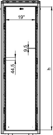
ÖN KAPAKSIZ GÖRÜNÜŞ
