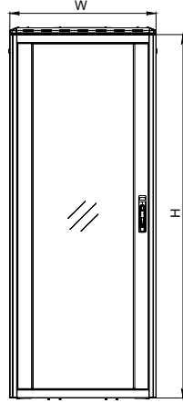
ÖN GÖRÜNÜŞ
