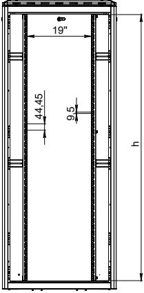
ÖN KAPAKSIZ GÖRÜNÜŞ
