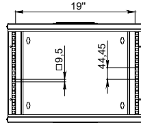
FRONT VIEW WITOUT DOOR
