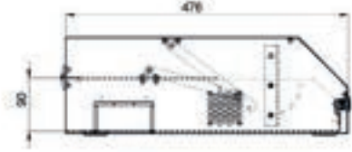
Yan Görünüş
