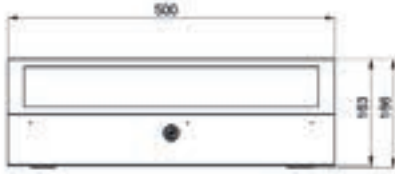
Ön Görünüş
