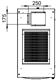
ÜST GÖRÜNÜŞ
