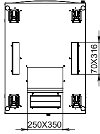
ALT GÖRÜNÜŞ
