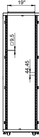
ÖN KAPAKSIZ GÖRÜNÜŞ
