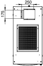
ÜST GÖRÜNÜŞ
