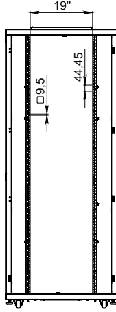
KAPAKSIZ ÖN GÖRÜNÜŞ
