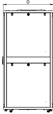
YAN GÖRÜNÜŞ
