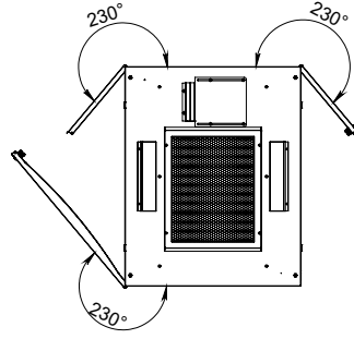
KAPI DÖNME AÇILARI
