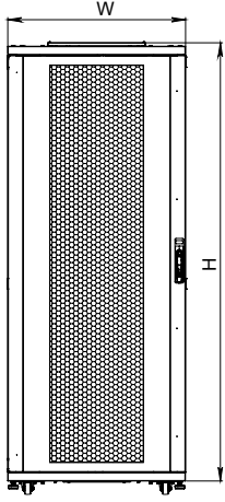
ÖN GÖRÜNÜŞ
