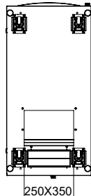
ALT GÖRÜNÜŞ
