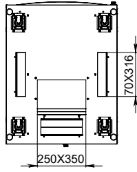
ALT GÖRÜNÜŞ
