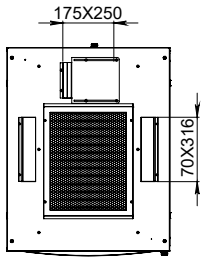
ÜST GÖRÜNÜŞ
