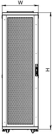
ÖN GÖRÜNÜŞ
