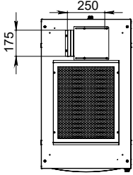
ÜST GÖRÜNÜŞ
