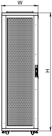
ÖN GÖRÜNÜŞ
