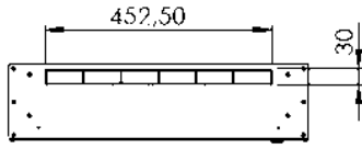
Üst Görünüş
