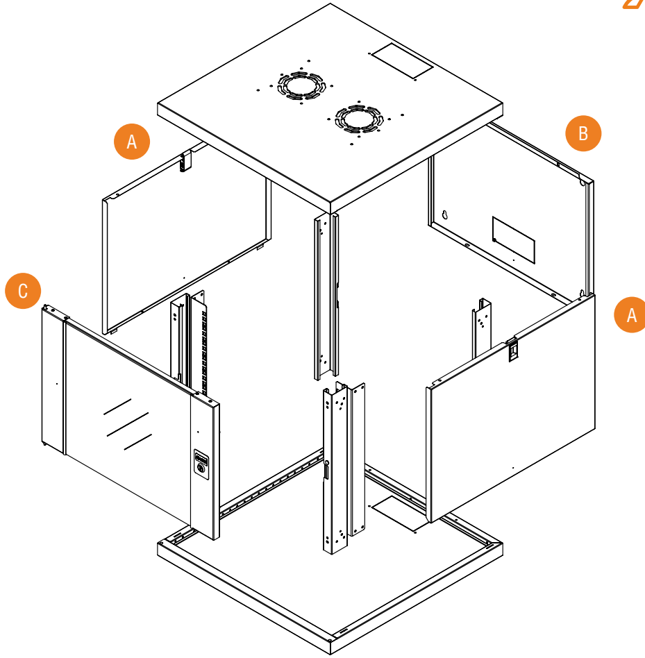
19" Ager Duvar Tipi AGENA FLAT Serisi
