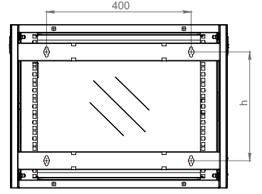
Arka Görünüş
