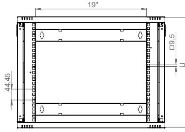
Ön Görünüş Cihaz Dikme Ölçüleri
