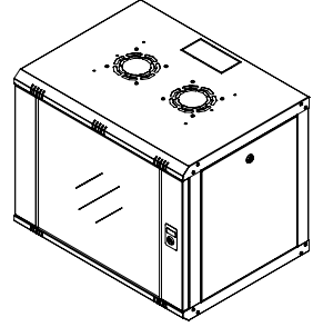
İZOMETRİK GÖRÜNÜŞ
